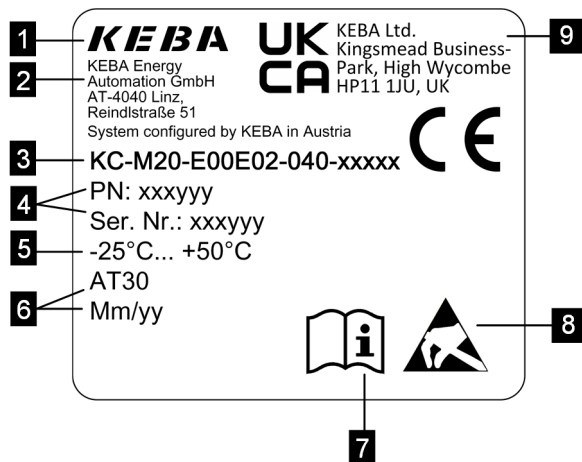
Fig. 3-8: Targhetta identificativa
