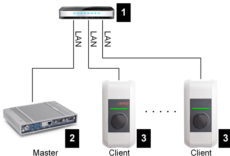
Fig. 2-5: Collegamento tramite router o switch
